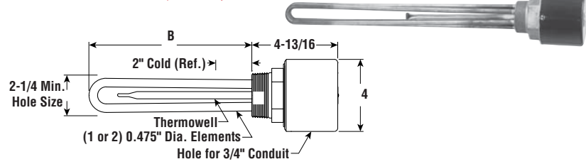
E2 — Dimensions (Inches)
